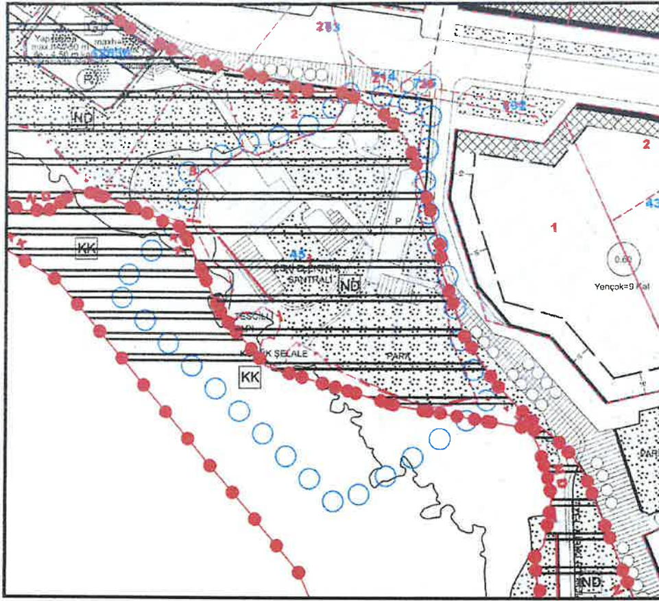
Plan 3: 1/1.000 Ölçekli Uygulama Planı
